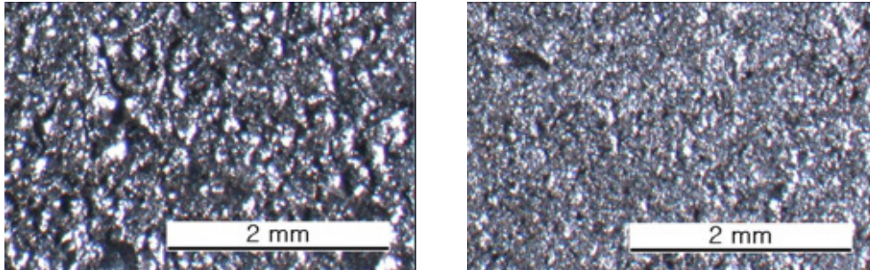
Perfil granallado con la granalla antigua Perfil granallado con Profilium
